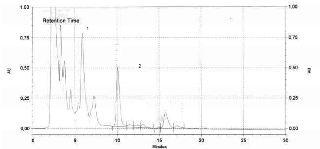
Σχήμα 6 — Χρωματογράφημα HPLC ασαπυνοποιητών υλών ελαιόλαδου διαχωρισμένων με HPLC με τη χρήση ανιχνευτή υπεριώδους. (1) Αλειφατικές και τριτερπενικές αλκοόλες (2) Στερόλες και τριτερπενικές διαλκοόλες.
